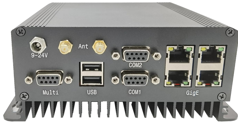
NANO-SYS-2006 背面接口指示图
